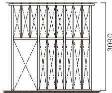
立面 (mm)
